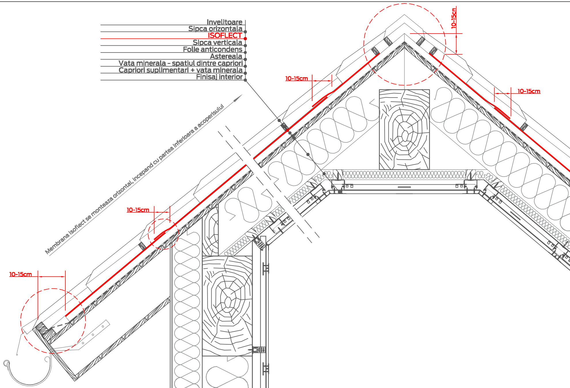
SILVER/BRONZE cu o singura sipca de apa Detaliu general
