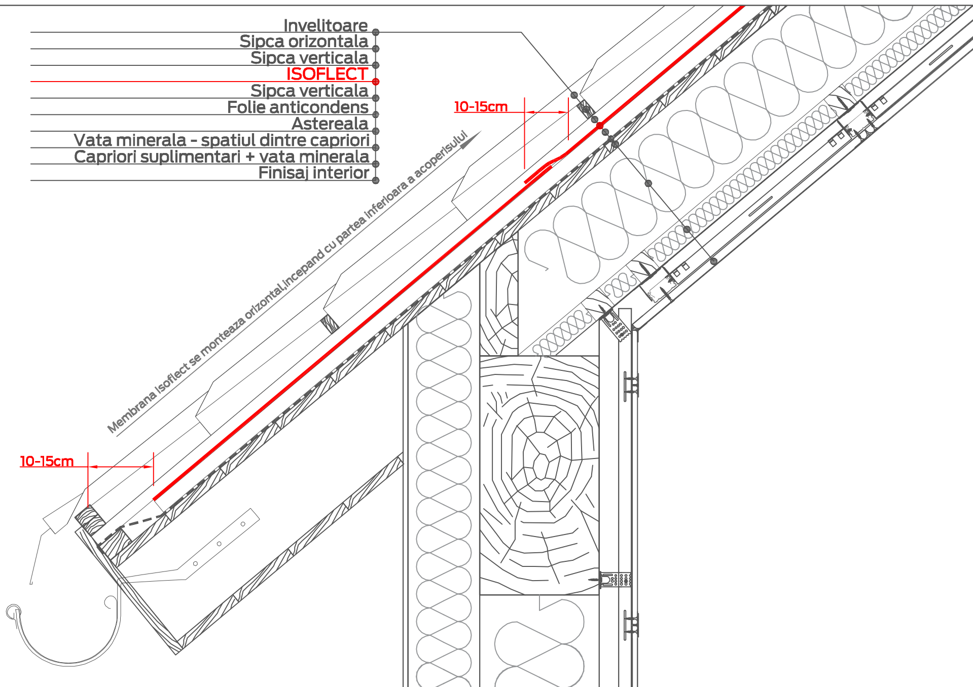
SILVER/BRONZE cu doua sipci de apa Detaliu streasina
