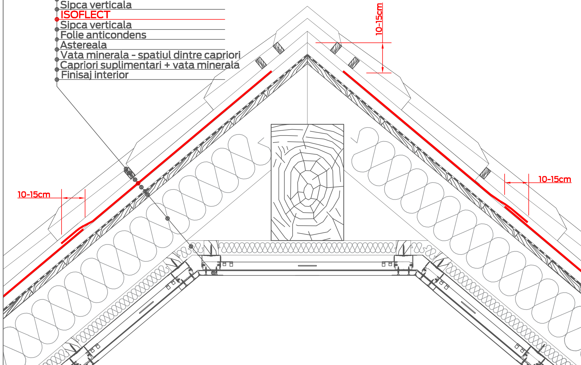
SILVER/BRONZE cu doua sipci de apa Detaliu coama
