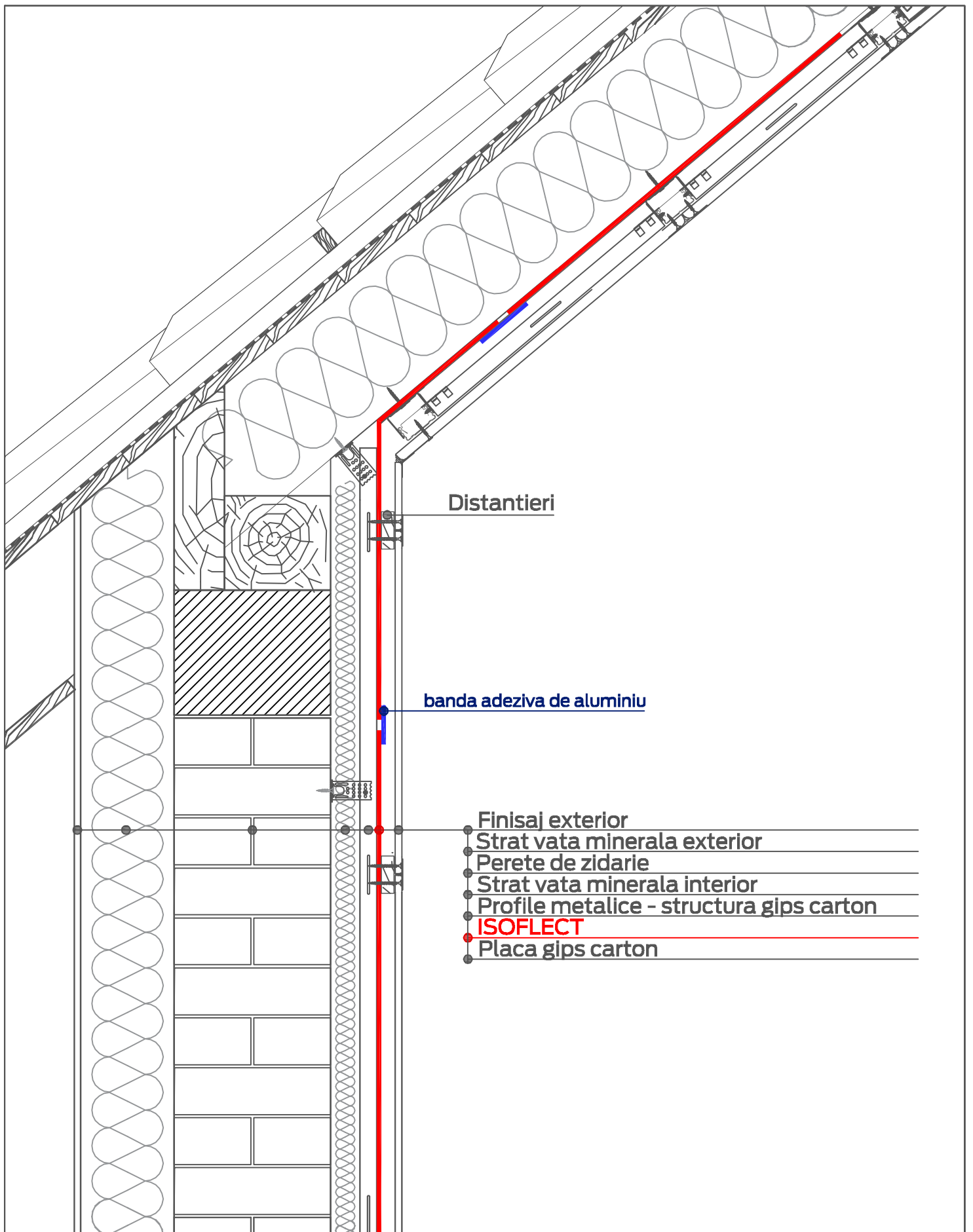
GOLD - detaliu perete interior pe structura de caramida
