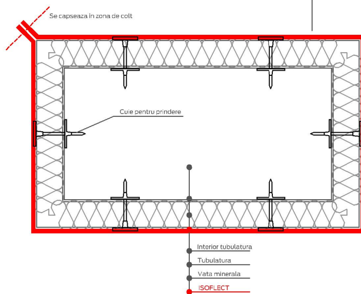
Sectiune transversala prin tubulatura
