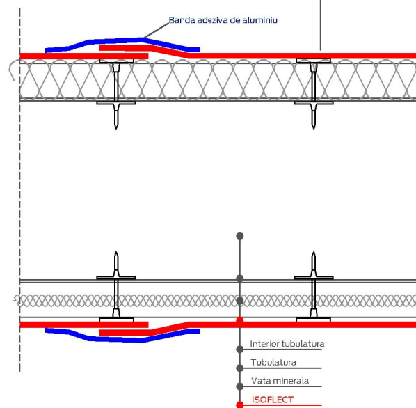
Sectiune longitudinala prin tubulatura
