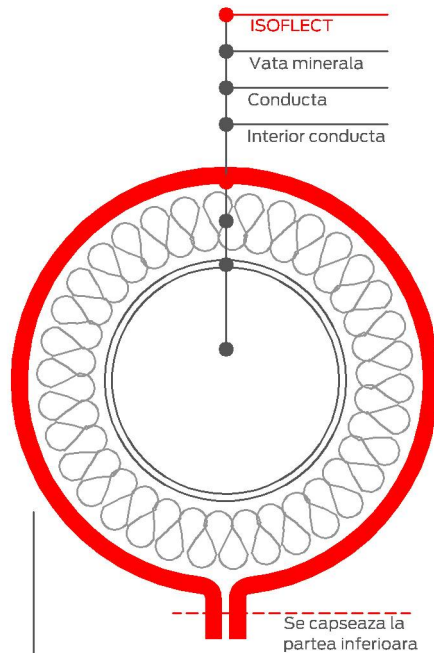
Sectiune transversala prin conducta
