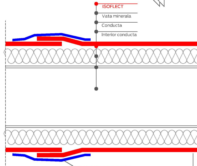
Sectiune longitudinalala prin conducta
